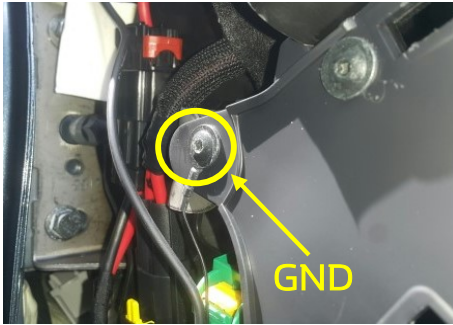
3. 운전석 사이드 커버와 퓨즈박스 커버를 분리해 퓨즈박스까지 전원선을 빼 주세요. 전원배선 중 적색선은 ACC에 검정색선은 GND(접지)에 연결해 주시면 됩니다.
