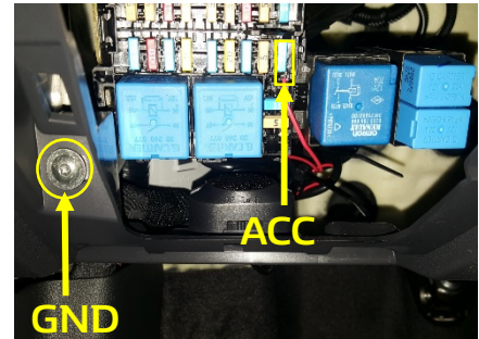
4. 전원배선 중 적색선은 ACC에 검정색선은 GND(접지)에 연결해 주시면 됩니다. (※ACC: 시가라이타 퓨즈)
